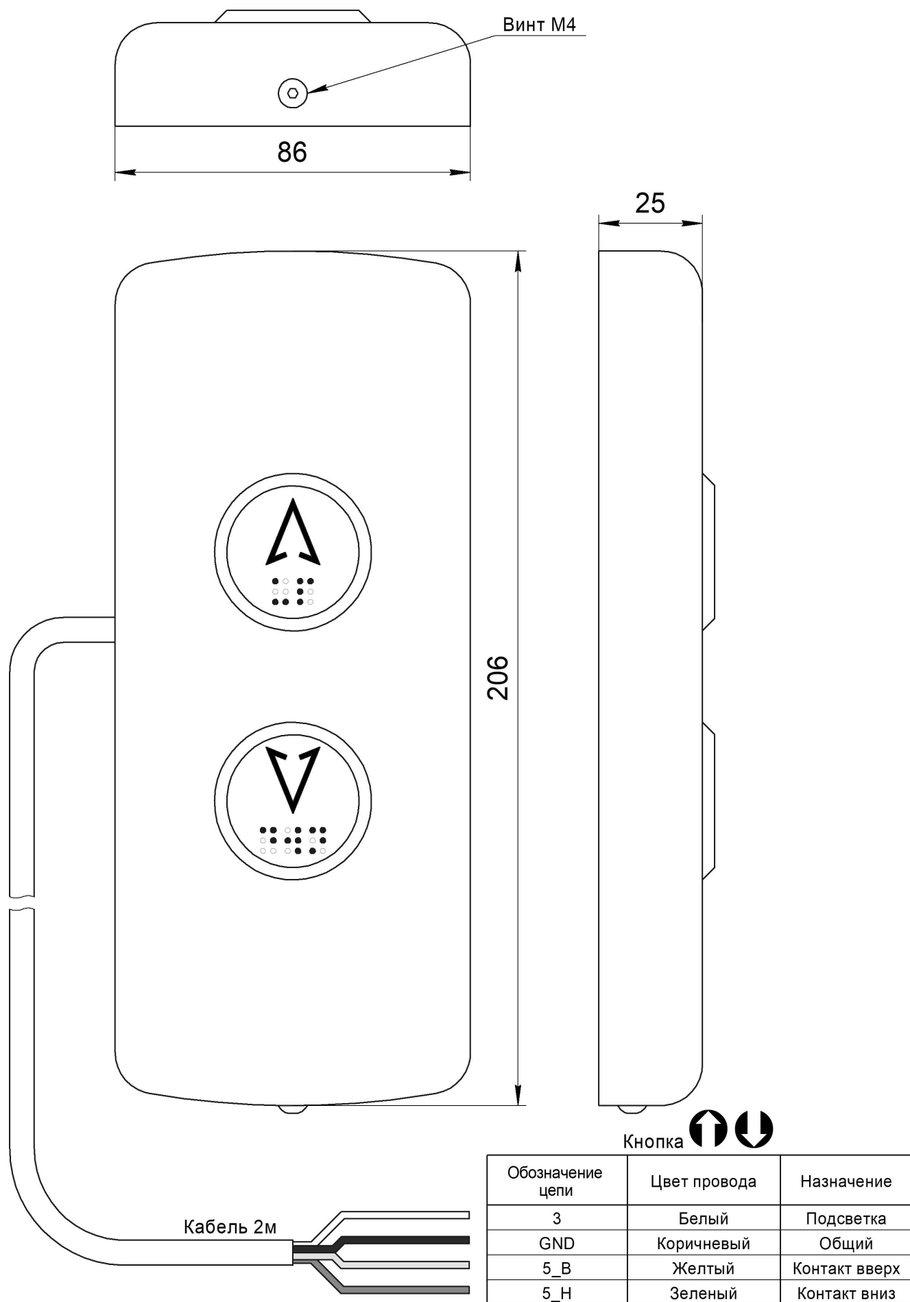
Рис.1 Внешний вид, габаритные и установочные размеры Вызывного поста ВП-2103-05
